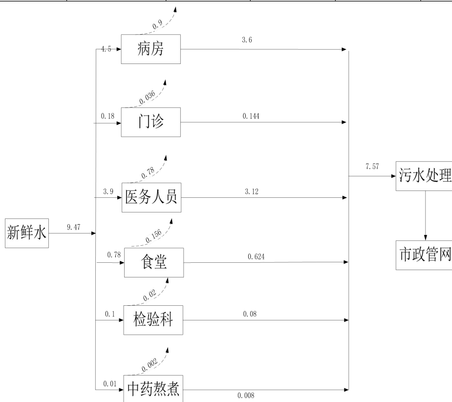
图 2.2-1 项目水平衡图 m 3 /d
