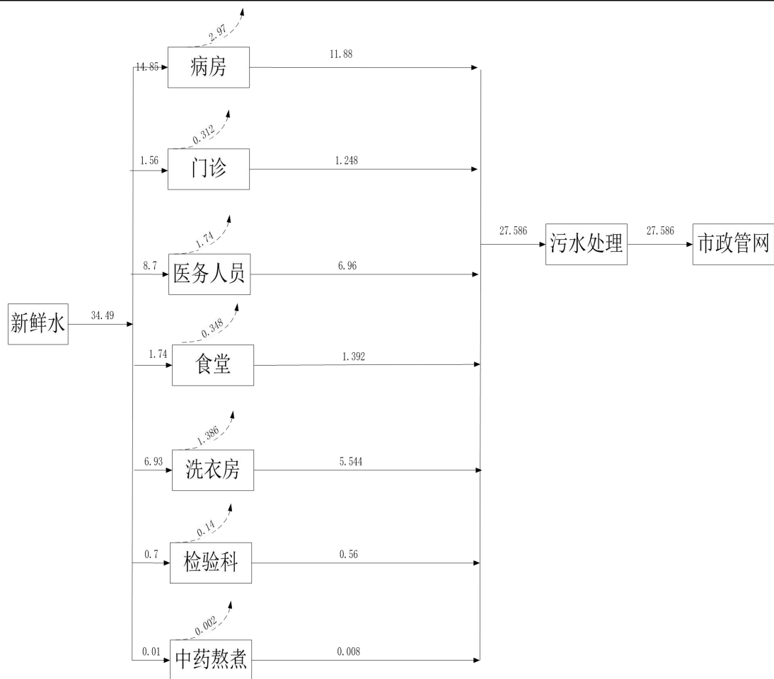
图 2.2-1 项目水平衡图 \text{m}^3/\text{d}
