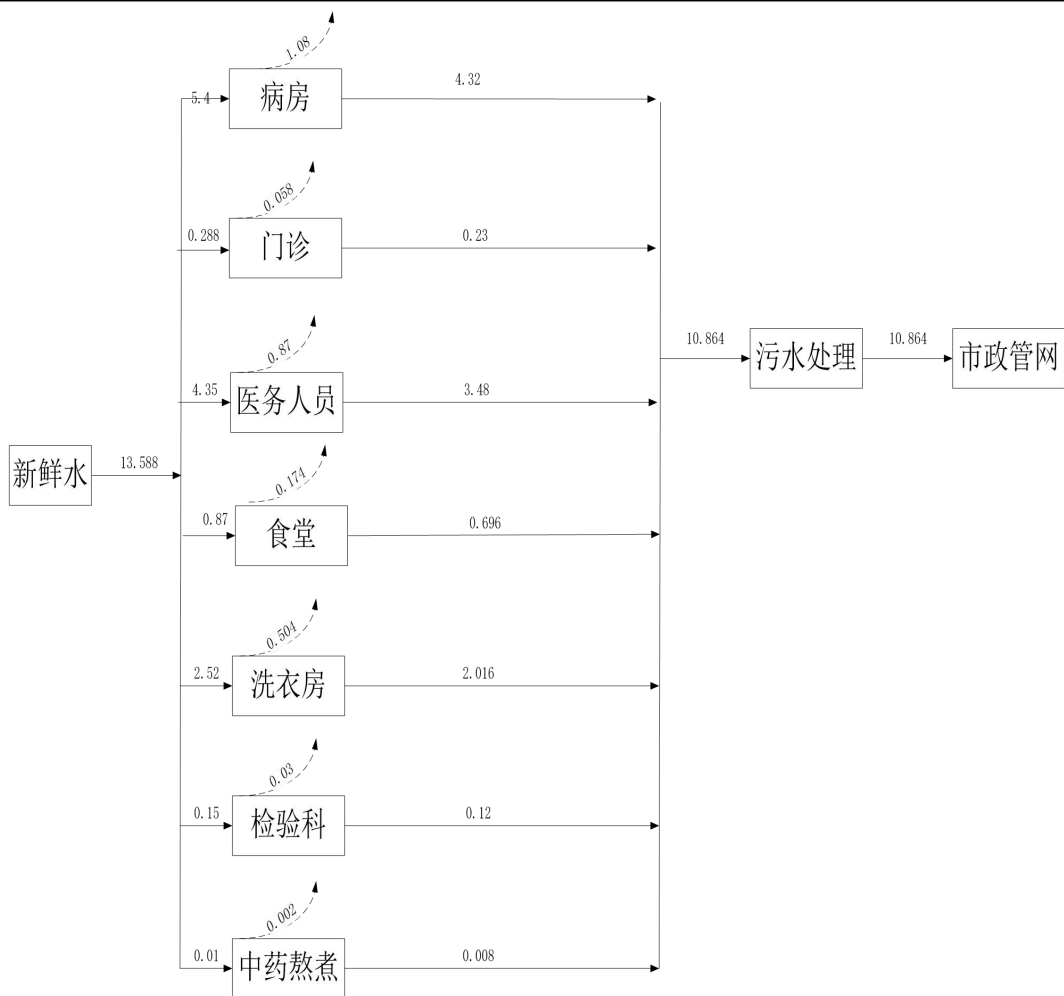
图 2.2-1 项目水平衡图 m³/d
