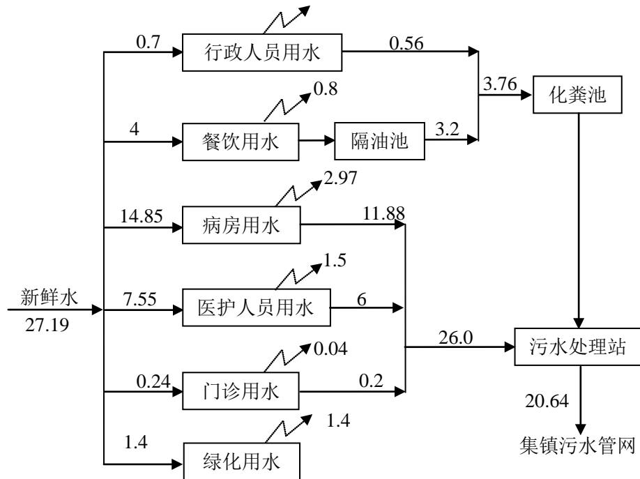
图 1-1 项目水平衡图 (单位: m 3 /d)
