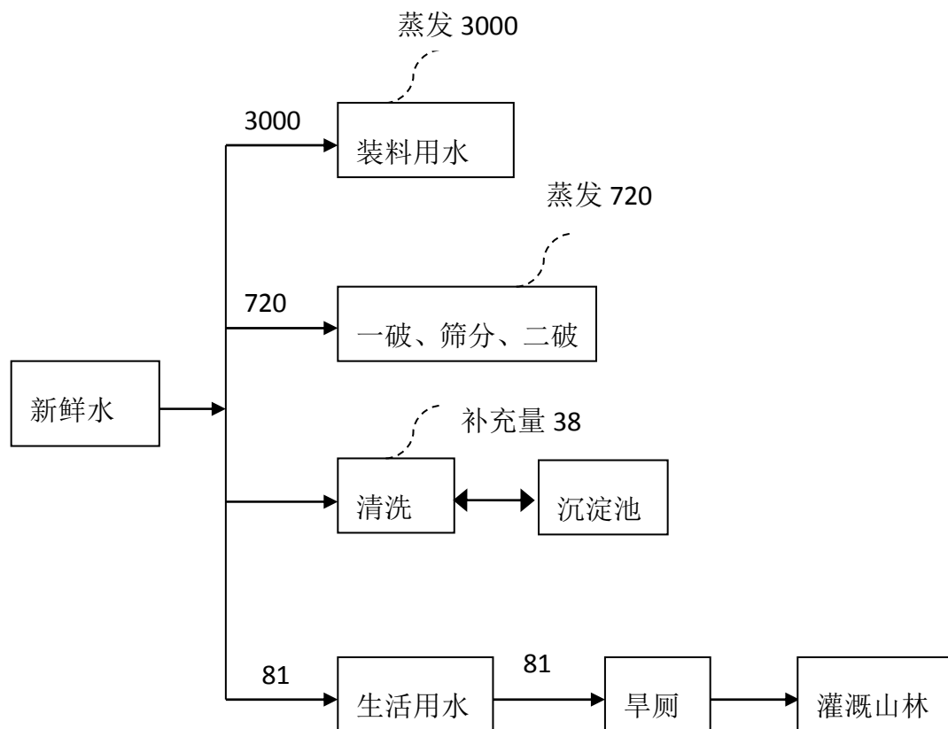
图 5-2 项目水平衡分析图 (t/a)
